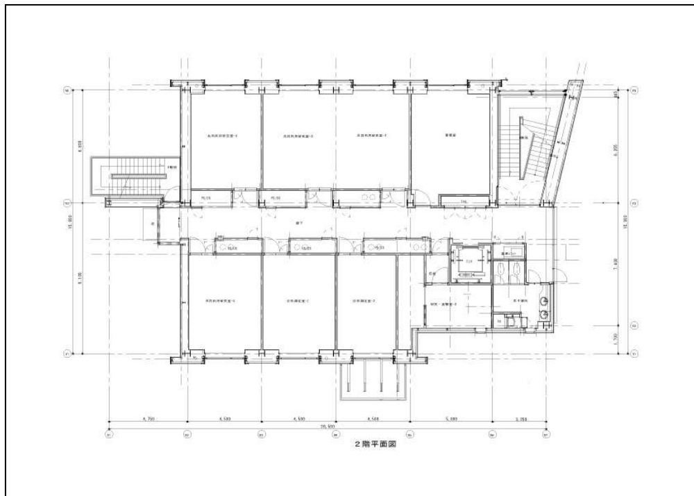
〔2 階平面図〕
